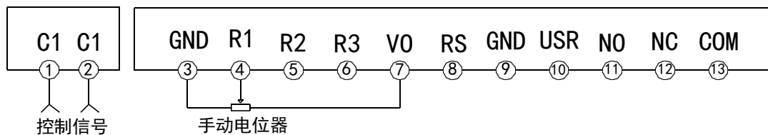
图 4: 手动接线图
