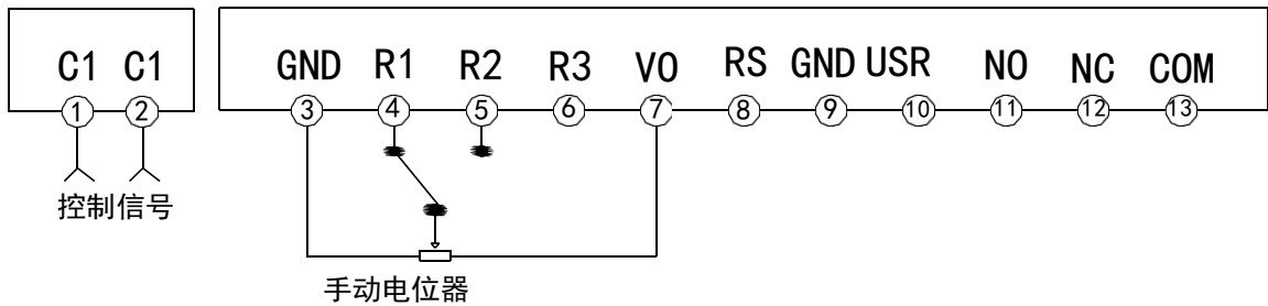
图 7：手动及自动组合接线图
