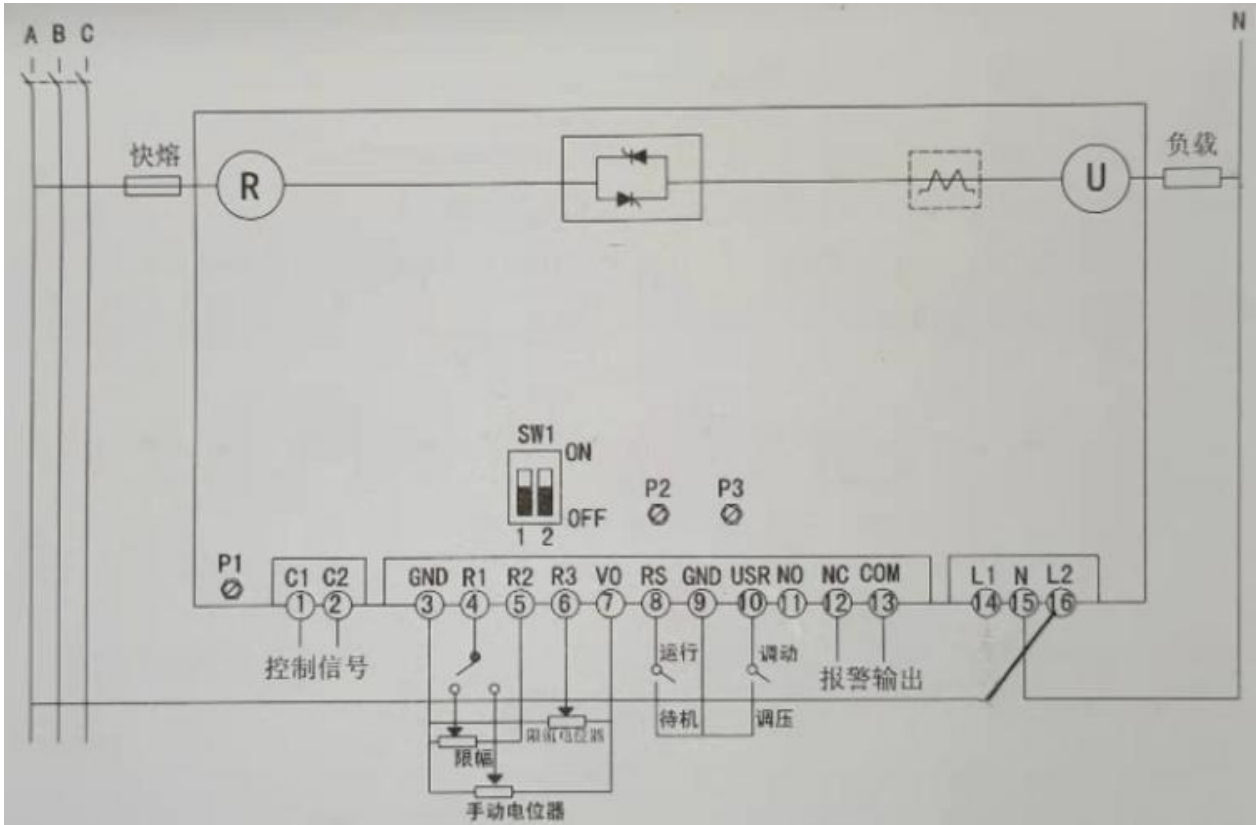
图 1 SP1B 整机完整接线图
